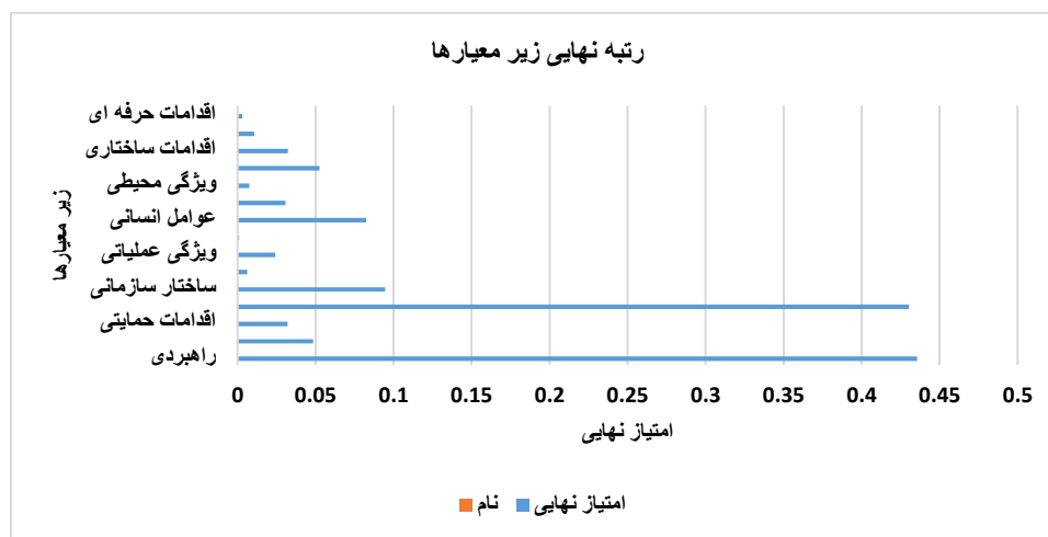
نمودار (۸): ضریب و امتیاز نهایی محاسبه شده برای گزینه‌ها بر اساس مدل AHP
